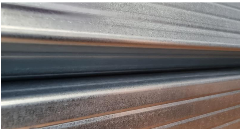
Rys. 1: Profile składowane na sucho – brak ryzyka wystąpienia białej rdzy.
